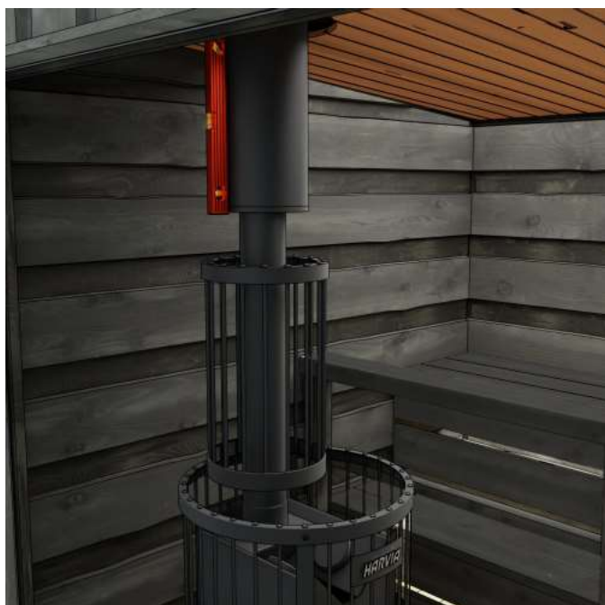
13. Controleer of de schoorsteen mooi recht staat. Verplaats indien nodig de kachel.
